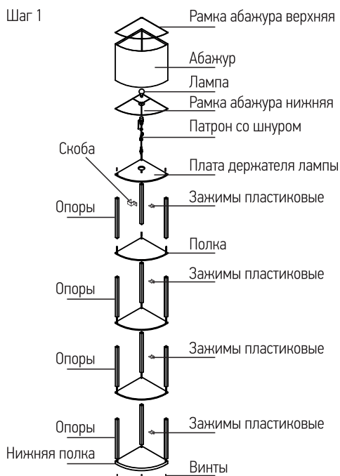
Рис. 1 Сборка светильника
