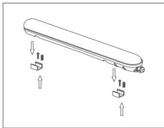
– Рисунок 1 – Установка при помощи монтажных скоб
